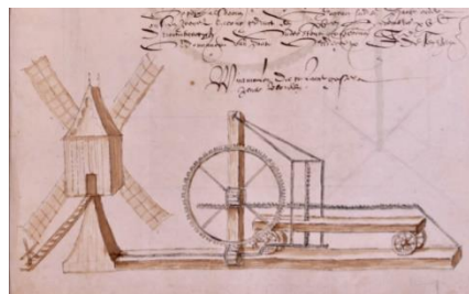
Illustratie bij de patentaanvraag uit 1593 bij de Staten van Holland en West-Friesland voor een door wind aangedreven zaagmolen door van Cornelis van Uitgeest. Foto Merlijn Hurx.
