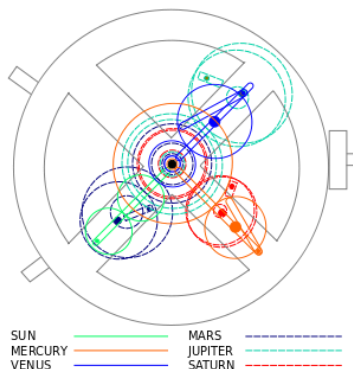
Voorblad en opstelling tandraden van het Antikythera mechanisme door Michael Wright.
